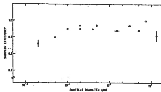
Figur 3 Insamlingseffektivitet som funktion av partikelstørlek.
