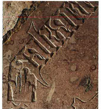
Detalj av Kämpestenen. I ytan kan man urskilja större delar av sjöiljor, stromatoporider och rugosa koraller; det mera finkorniga fyllningsmaterialet består till största delen av krossade sjöiljor. Fossilerna antyder att stenen brutits på södra delen av Gotland. Foto Thorsten Persson.
