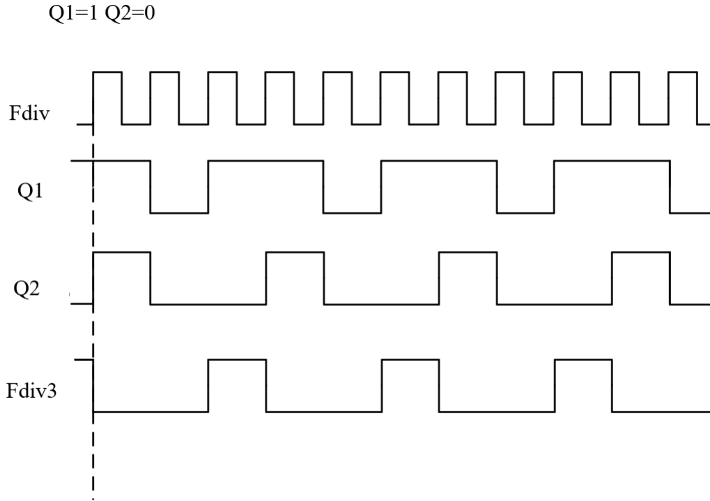
Figure 3.22: Q1Q2=’10’
