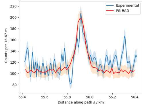
(d) “Road 3”, NaI(Tl) (gross counts)
